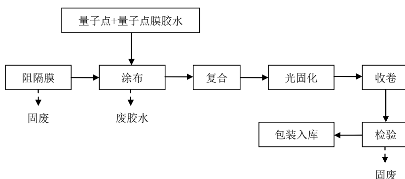
图 2.2-3 量子点膜生产工艺流程图
