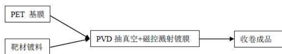
图 2.2-4 PVD 线生产工艺流程图
